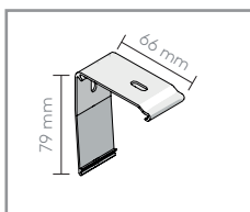
Universalträger 24.7511 für Wand und Decke
