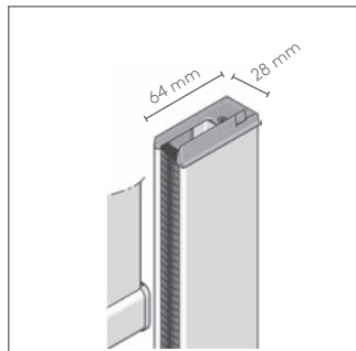
64 mm (Standard) Stoff und Unterleiste sind seitengeführt
