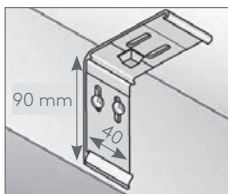
Universälträger für Wand und Decke
