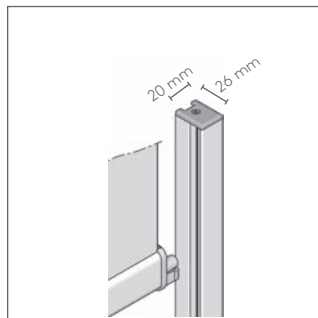
20 mm nur Unterleiste ist seitengeführt
